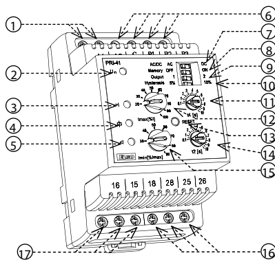
Descrierea comutatorului DIP
